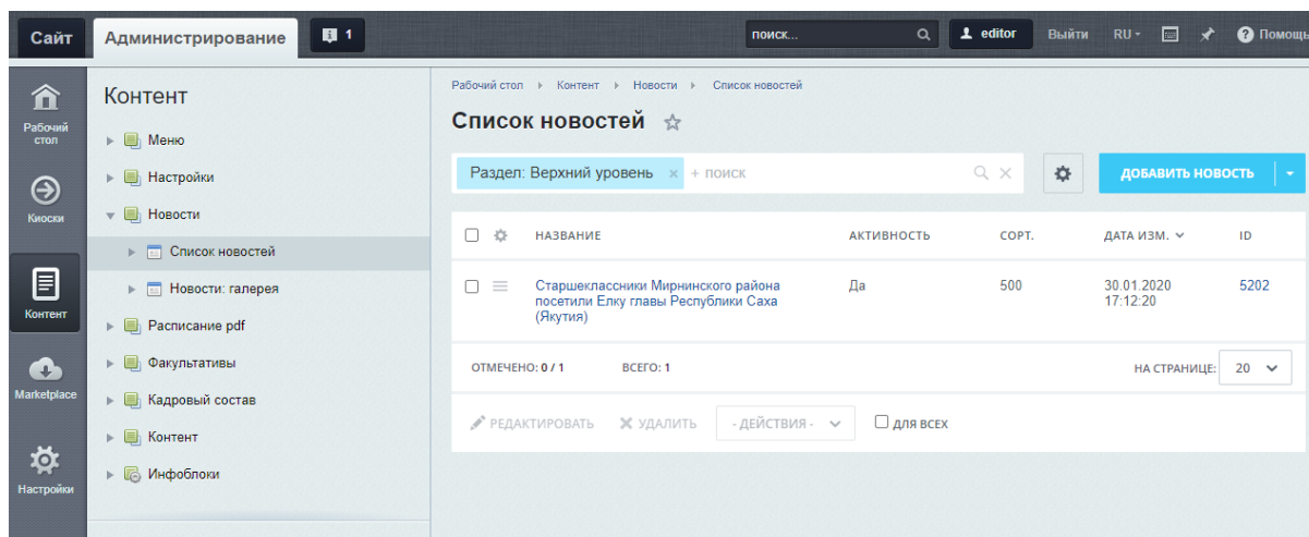
Рис. 6. Список новостей
